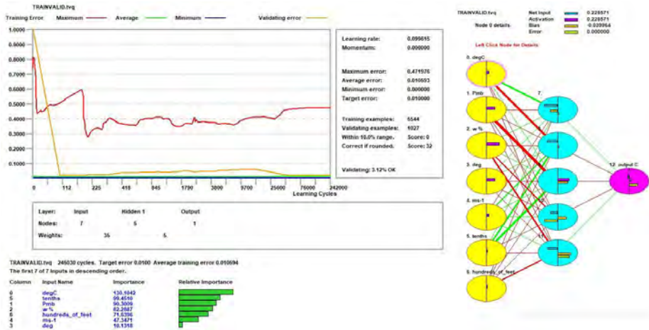
Figura 3: Addestramento Rete Belgio
