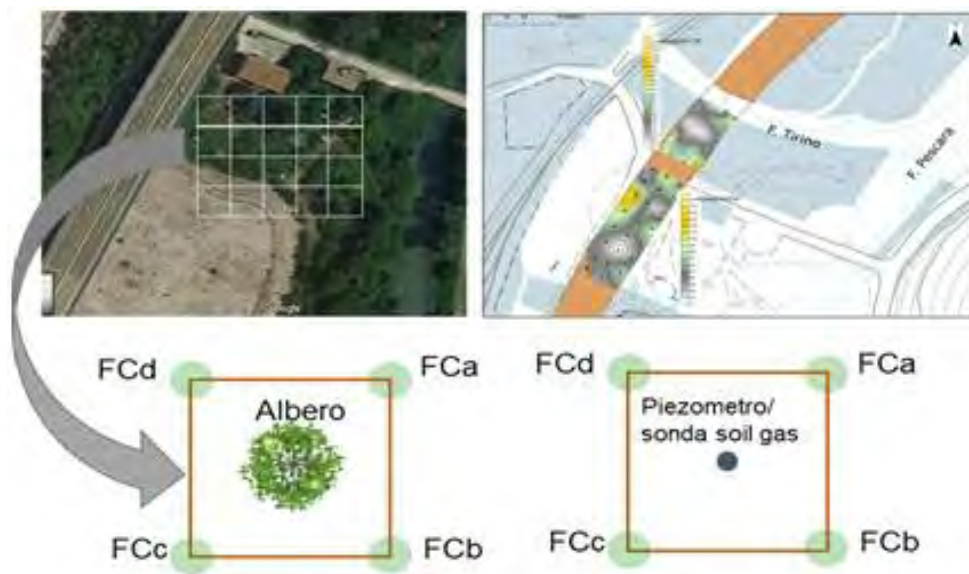
Figura 3: Utilizzo integrato di camere di flusso e phytoscreening
