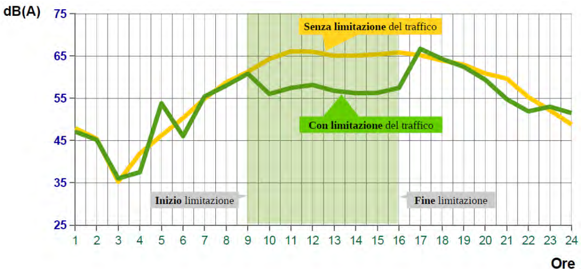
Figura 2: Confronto fra i livelli di rumore medi orari rilevati durante i giorni di normale apertura al traffico (linea "gialla") e quelli rilevati nei mercoledì di limitazione del traffico (linea "verde")
