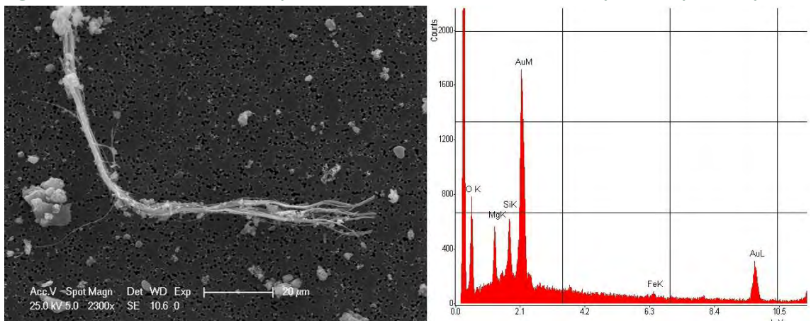
Figura 4: Fascio di crisotilo al microscopio elettronico a scansione (SEM) e relativo spettro da spettroscopia EDX
