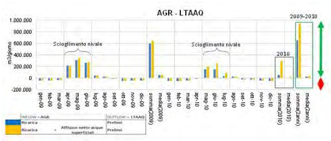
Figura 2: Andamento temporale della differenza tra ricarica netta dell'acquifero (AGR) e prelievi (LTAQ)
