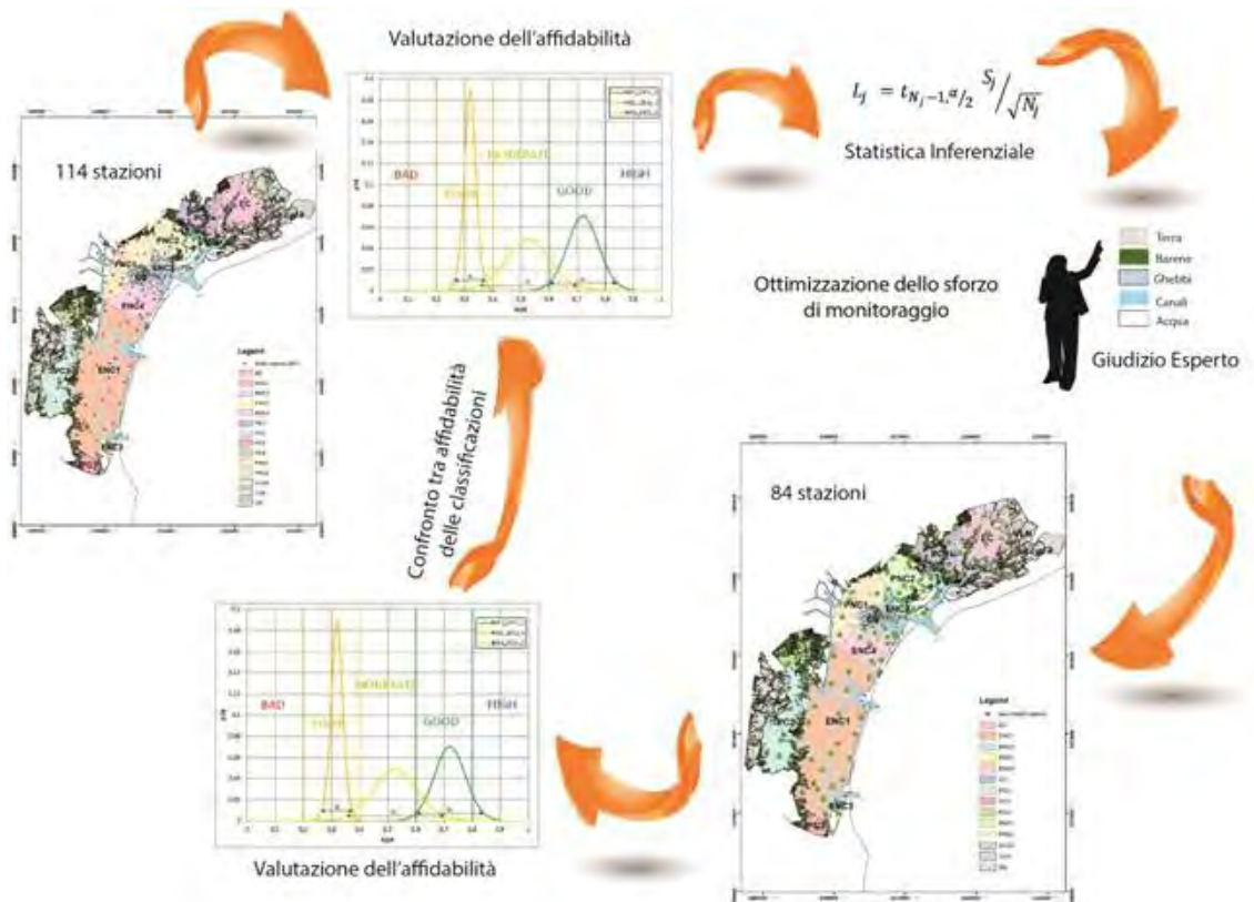
Figura 1: Schematizzazione dell'Approccio Multiplo per la verifica dell'affidabilità della classificazione e per l'ottimizzazione dello sforzo di monitoraggio applicato alla Laguna di Venezia
