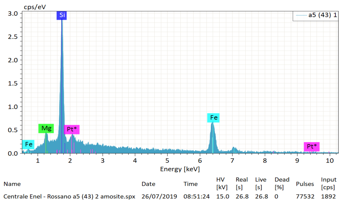
Figura 8 – Spettro di Amosite
