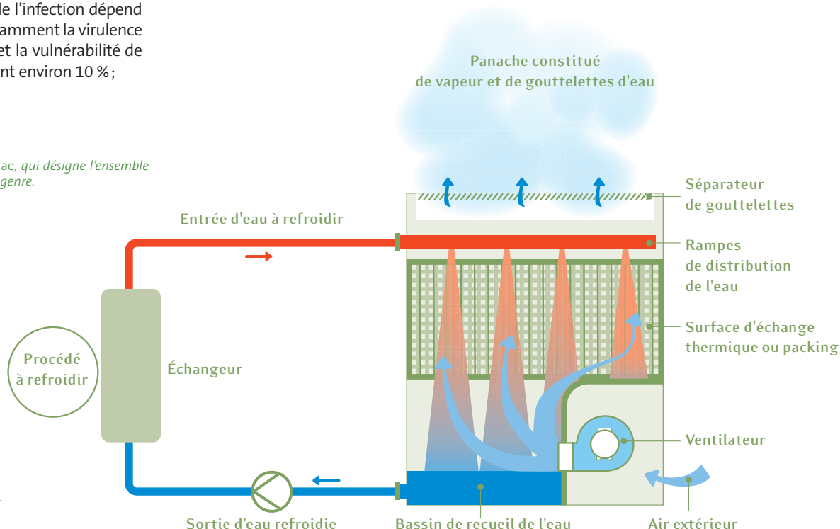
Figure 1. Schéma d'une tour aéroréfrigérante de type humide
