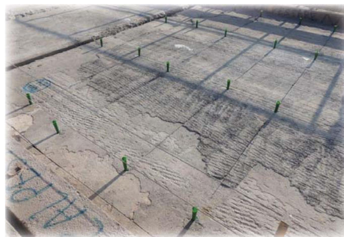
La carreggiata Sud a lavori di predisposizione per l'abbattimento completati. I coni verdi sono inseriti nei fori da mina. Tra i fori da mina la soletta tagliata a disco diamantato.
