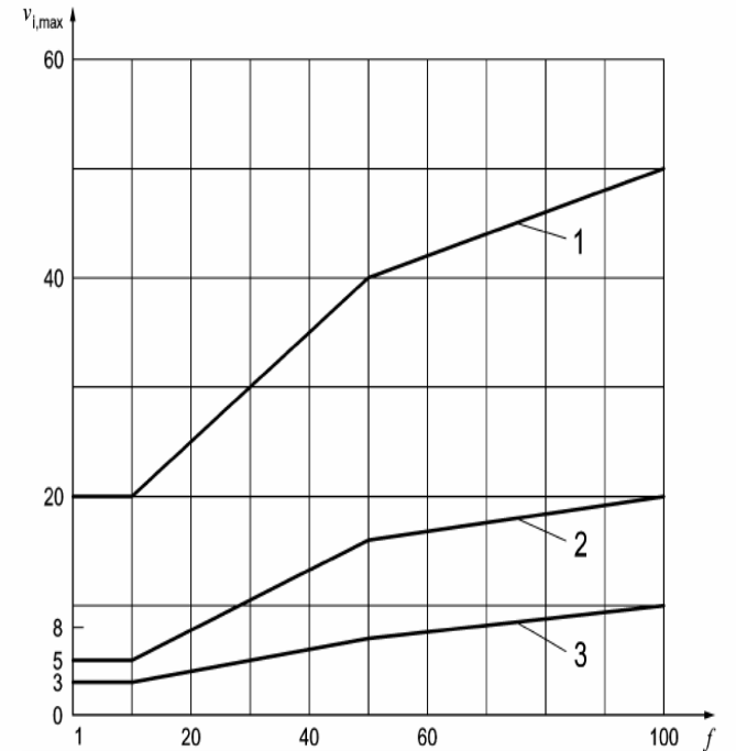
Bild 1 Graphische Darstellung der Fundament-nhaltswerte von Tabelle 1 Rappresentazione grafica dei valori di riferimento in tabella 1 (delle DIN 4150-3)
